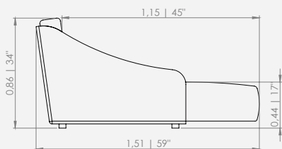
Módulo aberto
