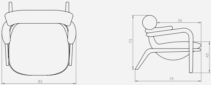
Configurações de Poltrona Poltrona 82 - 1ass(82 x 79)
