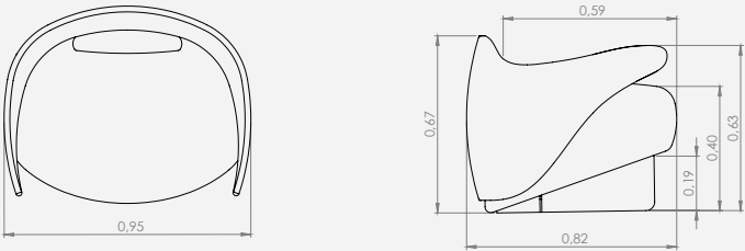
Configuração de Poltrona Poltrona 95 - 1ass(81) + 2br(7) + 1alm/rim(45x23)
