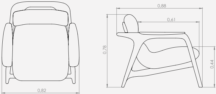
Configurações de Poltrona Poltrona 82- 1ass(61 x 61)
