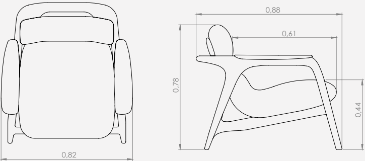
Configurações de Poltrona Poltrona 82- 1ass(61 x 61)
