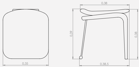
Configurações de Banco Cadeira 35 - 1ass(35 x 38)
