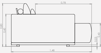
Módulo aberto
