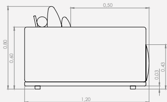
Módulo fechado
